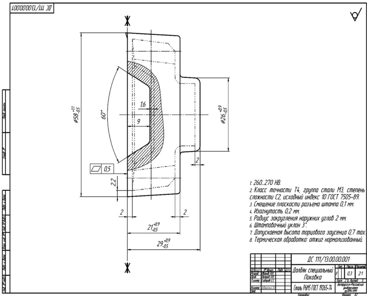
Рисунок 1 – Чертеж поковки
