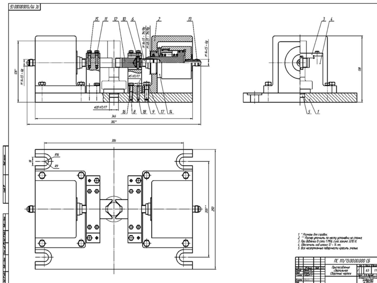
Рисунок 4 – Чертеж станочного приспособления
