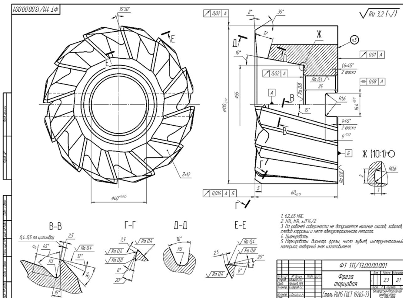
Рисунок 2 – Чертеж инструмента
