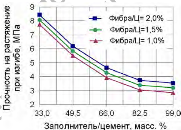
Рисунок 4 – Характер изменения прочности фибробетона в зависимости от содержания микросфер и фибры («Виннапас»/Ц=8 %)
