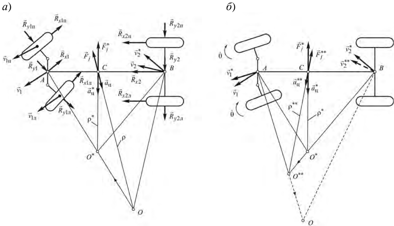
Рисунок 1 – Схема заноса заднего моста автомобиля при движении на повороте
