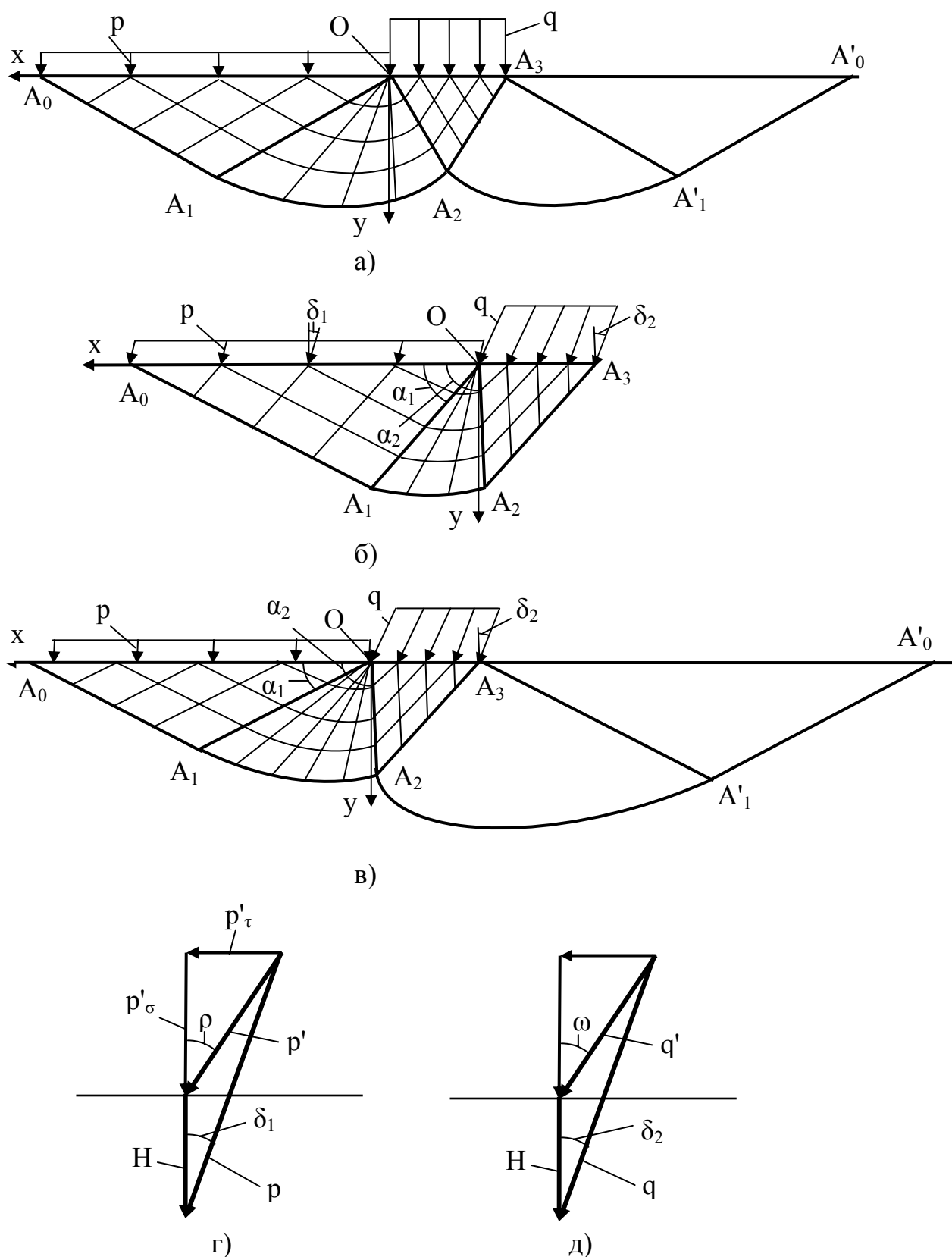
Рис. 1. Расчетные схемы разрушения грунта неподвижным отвалом (а), подвижным отвалом при движущейся (б) и неподвижной (в) призме волочения и схемы для расчета давлений на поверхность грунта при движущейся призме волочения (г) и движущемся ноже (д).
