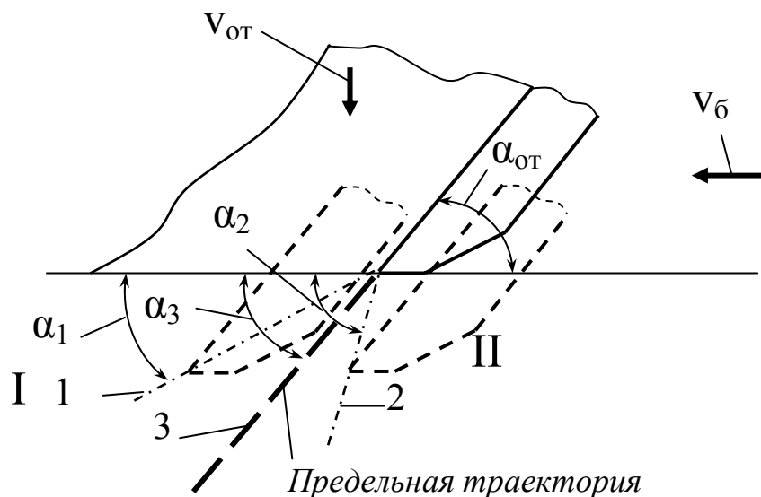
Рис. 2. Схема к расчету предельной траектории заглубления отвала.
