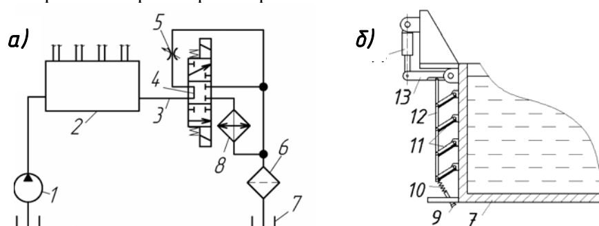
Рисунок - 2 Система подогрева рабочей жидкости основанная на уменьшении теплоотдачи гидробака машины: а – гидросхема системы подогрева; б – механическая схема гидробака
