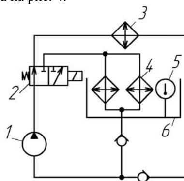
Рисунок - 4. Система подогрева гидравлического масла за счёт тепла охлаждающей жидкости двигателя внутреннего сгорания
