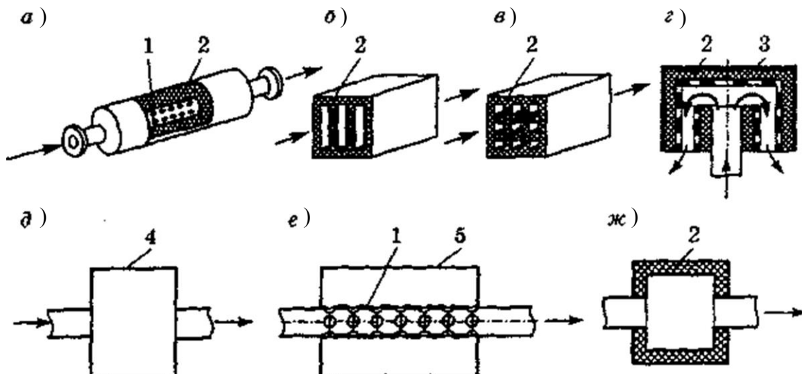
а – абсорбционного трубчатого типа; б, в – абсорбционного сотового типа; г – абсорбционного экранного типа; д, е – реактивного камерного типа; ж – комбинированного типа; 1 – перфорированные трубки; 2 – звукопоглощающий материал; 3 – стеклоткань; 4 – расширительная камера; 5 – резонансная камера
