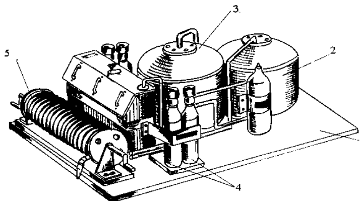
1 – рама; 2 – емкость для порошка; 3 – емкость для водного раствора; 4 – баллоны с азотом; 5 – катушка с пожарным рукавом
