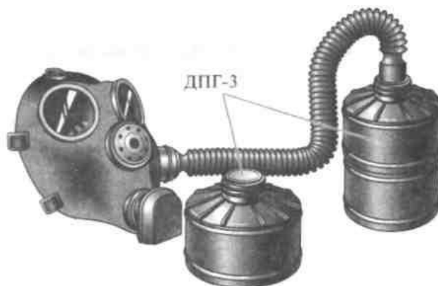
Рисунок 2.5 – Противогаз ГП-7 с дополнительным патроном ДПГ
