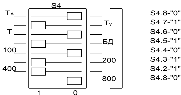
Рисунок 2.8 – Схема расположения движков кодового переключателя для измерений загрязненности поверхностей бета-излучающими радионуклидами
