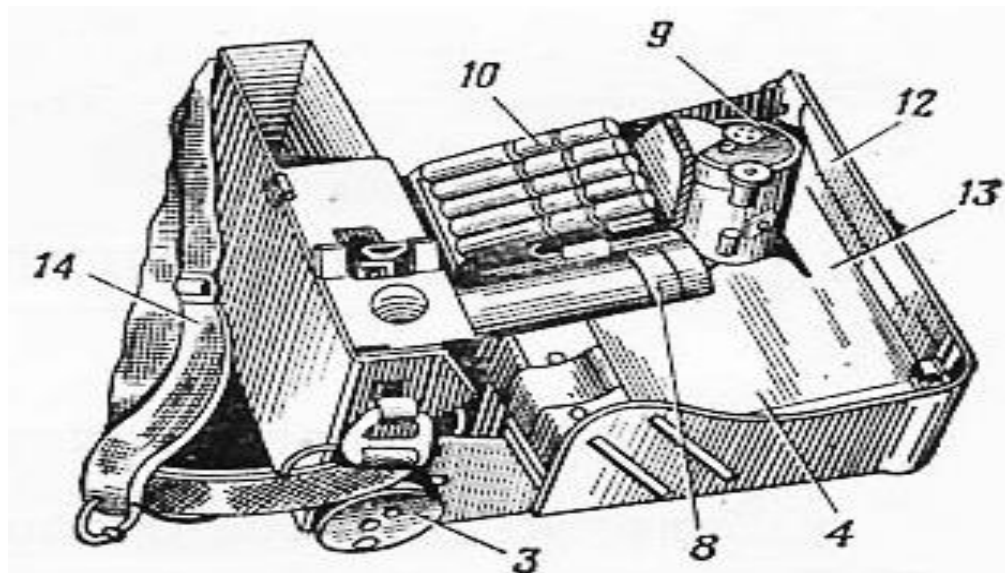
Рисунок 1.2 – Конструкция ВПХР
