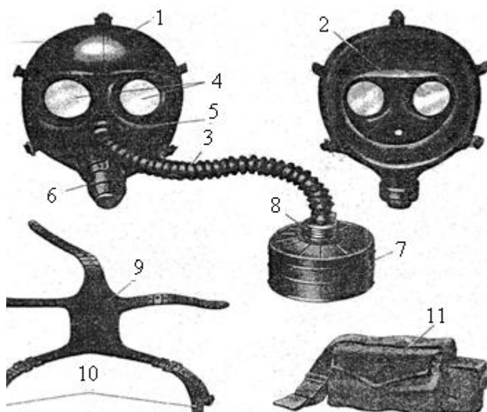
Рисунок 2.4 – Противогаз детский фильтрующий ПДФ-2Д
