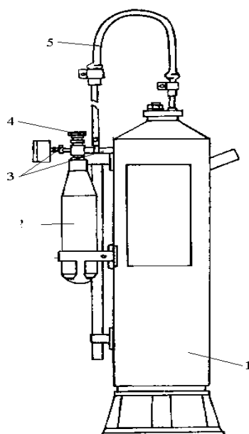
Рисунок 3.4 – Огнетушитель ОПС-10
