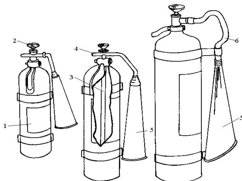
1 – баллон; 2 – вентиль; 3 – сифонная трубка; 4 – мембрана; 5 – раструб; 6 – гибкий шланг Рисунок 3. 3 – Схемы огнетушителей углекислотных ОУ-2, ОУ-5, ОУ-8
