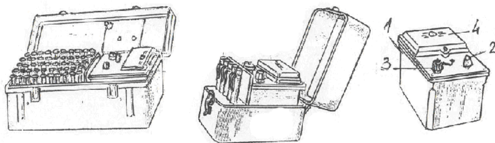
Рисунок – 1.3 Комплект дозиметров ДП-22В (ДП-24)
