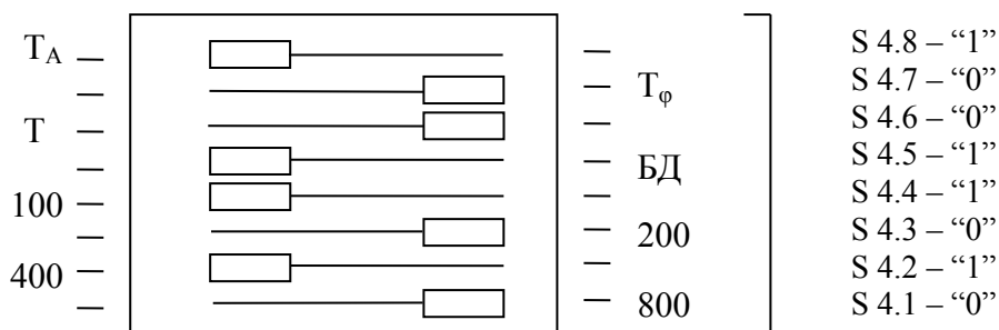
Рисунок 3.9 – Положения движков кодового переключателя S4
