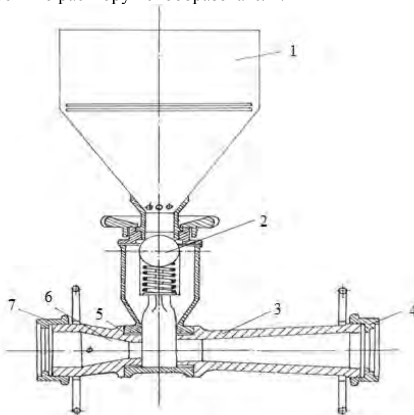
Рисунок 3.2 – Пеногенератор ПГ-50
