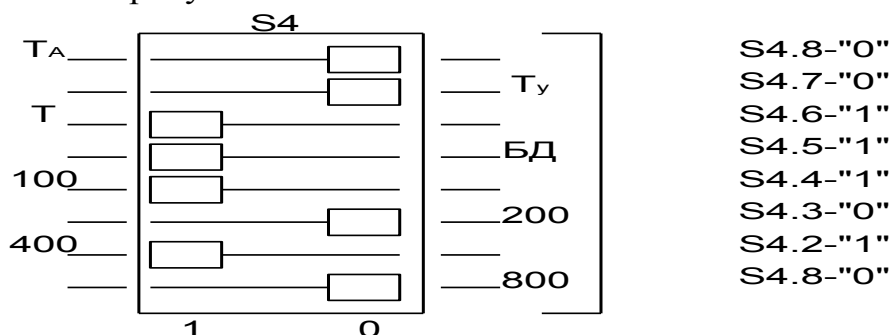
Рисунок 2.7 –Схема расположения движков кодового переключателя для измерения мощности полевой эквивалентной дозы \gamma -излучения в мкЗв/ч (мощности экспозиционной дозы \gamma -излучения в мкР/ч)
