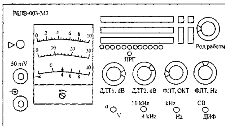
Рисунок 1.4 – Передняя панель прибора
