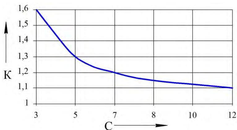
Рисунок 2.1 – Зависимость коэффициента K от индекса пружины
