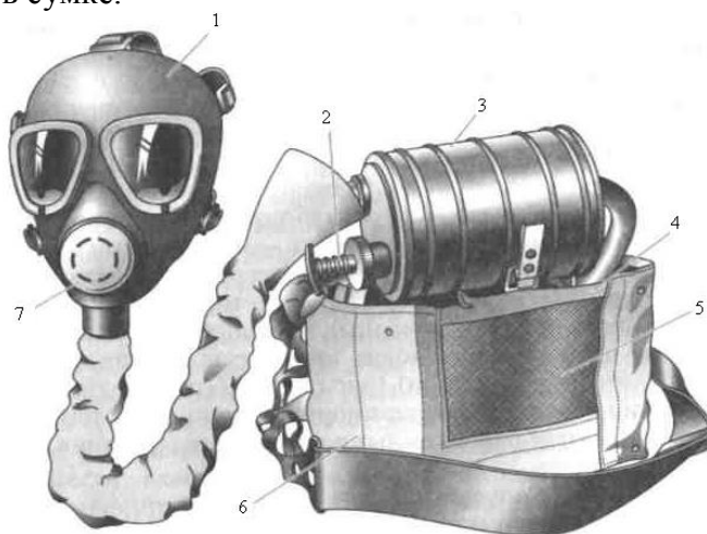
1 – маска МИА-1; 2 – пусковое приспособление; 3 – регенеративный патрон; 4 – каркас; 5 – дыхательный мешок; 6 – сумка; 7 – переговорное устройство
