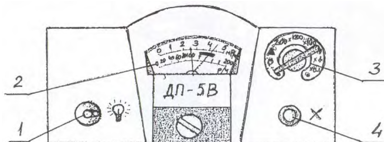
Рисунок 1.2 – Измерительный пульт
