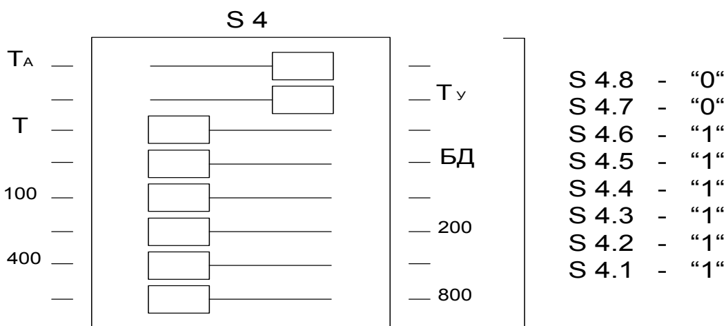
Рисунок 2.6 – Схема установки движков кодового переключателя для проверки работоспособности измерительной схемы прибора
