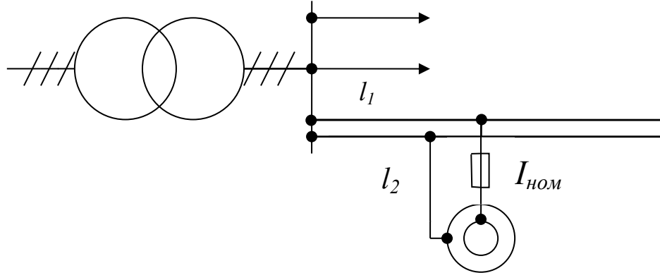
Рисунок 2.1 – Расчетная схема зануления
