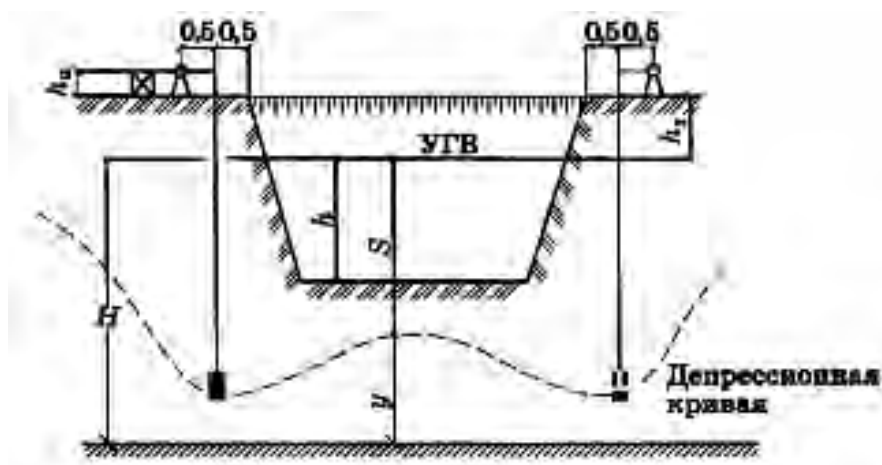
Рисунок 3 – Схема разреза котлована с установленными иглофильтрами
