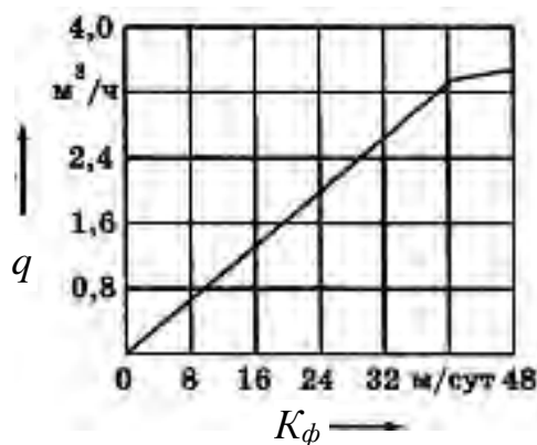
Рисунок 2 – Предельно допустимый дебит одного иглофильтра в зависимости от коэффициента фильтрации водоносного слоя
