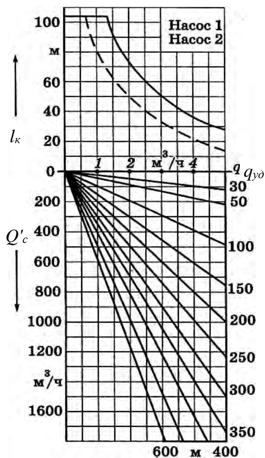
Рисунок 1 – График предельной длины всасывающего коллектора на один насосный агрегат ЛИУ-6
