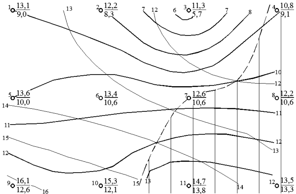
Рисунок 7.1 – Карта гидроизогипс
