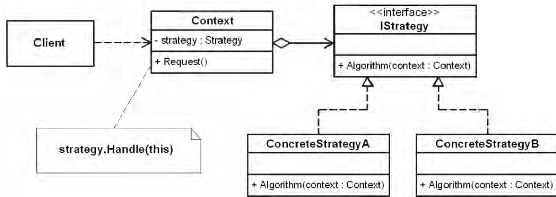
Рисунок 8.3 – Диаграмма классов шаблона Стратегия
