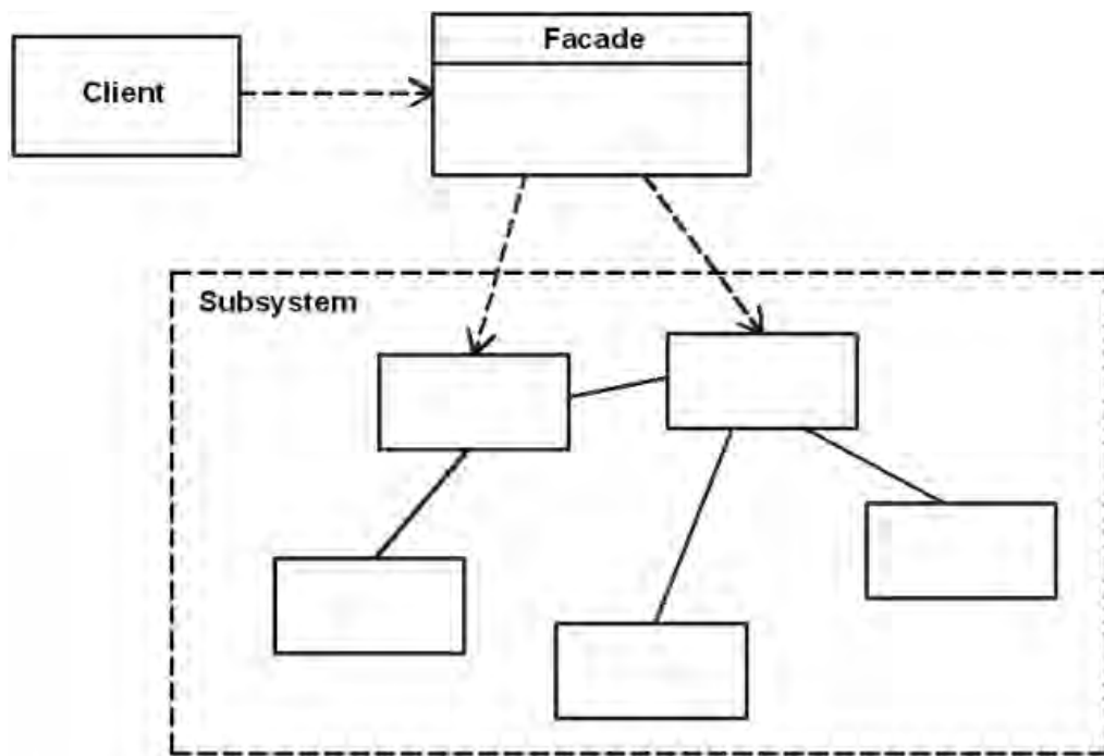
Рисунок 7.3 – Диаграмма классов шаблона Фасад
