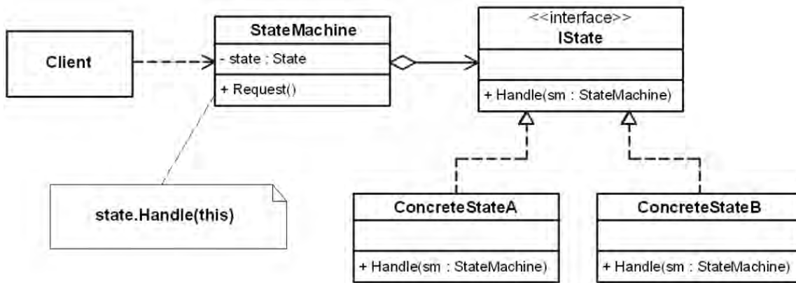
Рисунок 8.2 – Диаграмма классов шаблона Состояние
