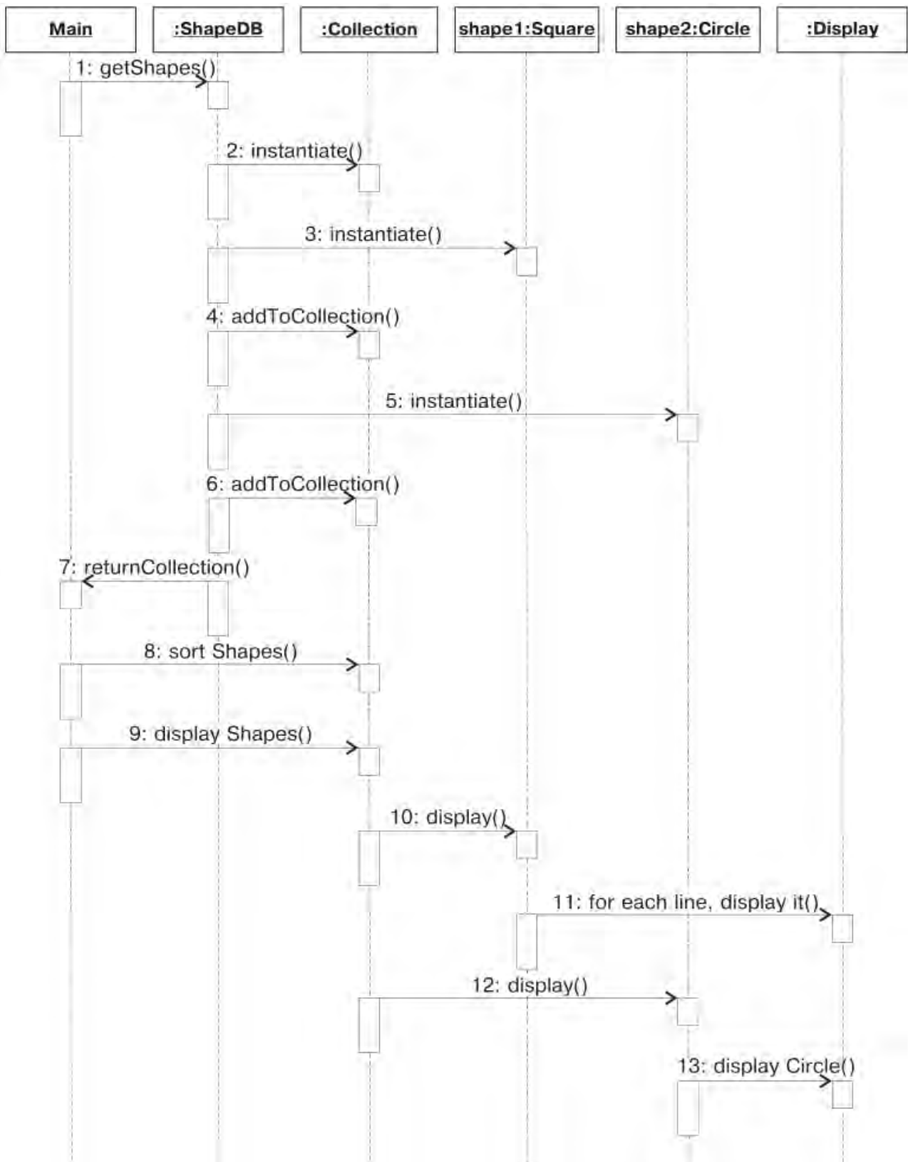
Рисунок 3.1 – Диаграмма последовательностей для программы обработки фигур
