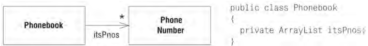
Рисунок 2.4 – Ассоциация «один ко-многим»
