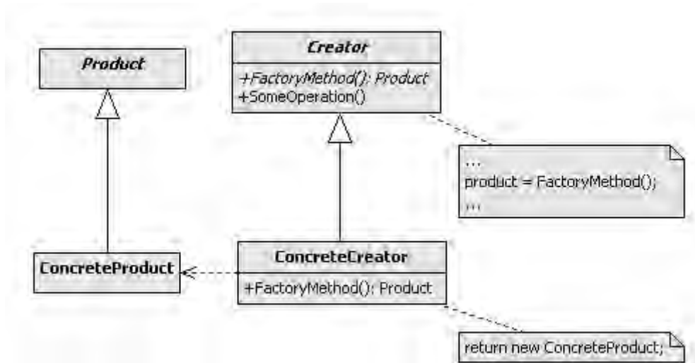
Рисунок 6.2 – UML-диаграмма шаблона Фабричный метод
