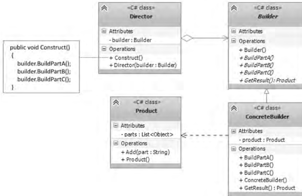
Рисунок 6.3 – UML-диаграмма шаблона Строитель
