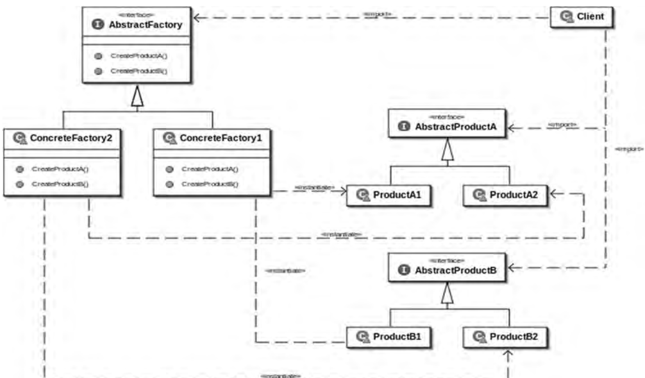
Рисунок 6.1 – UML-диаграмма шаблона Абстрактный продукт
