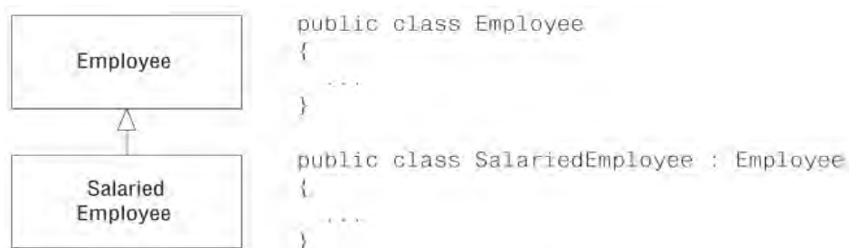
Рисунок 2.5 – Наследование
