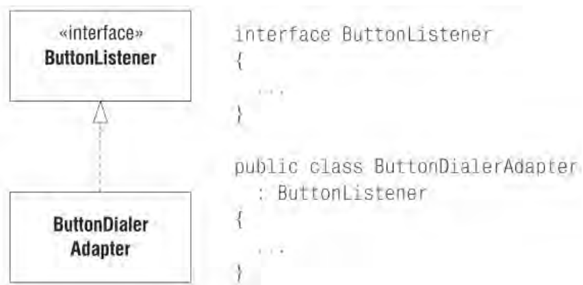
Рисунок 2.6 – Отношение «реализует»
