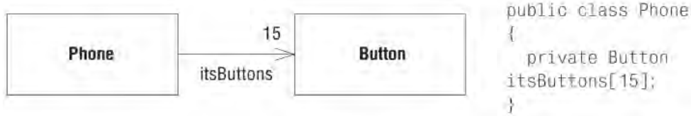
Рисунок 2.3 – Ассоциация
