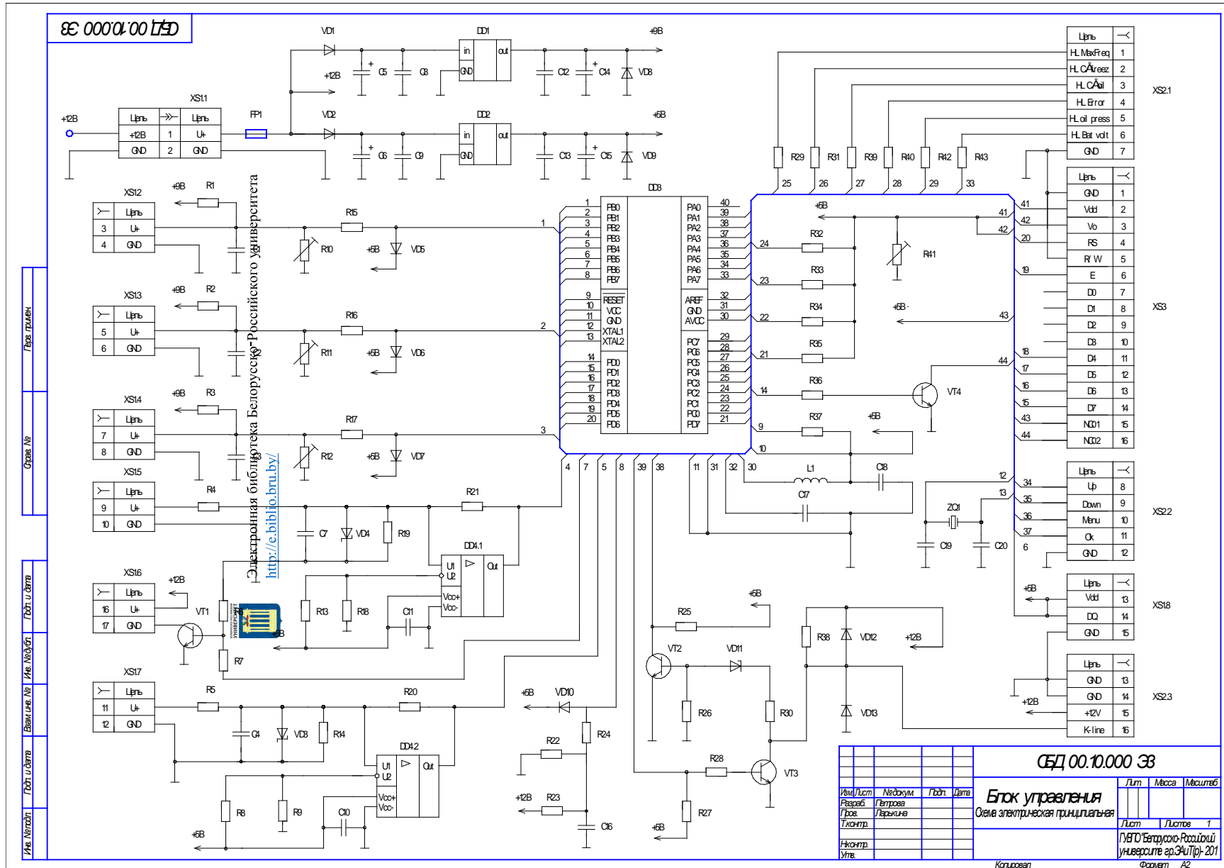
Рисунок В.6 – Пример выполнения чертежа схемы электрической принципиальной блока электронного
