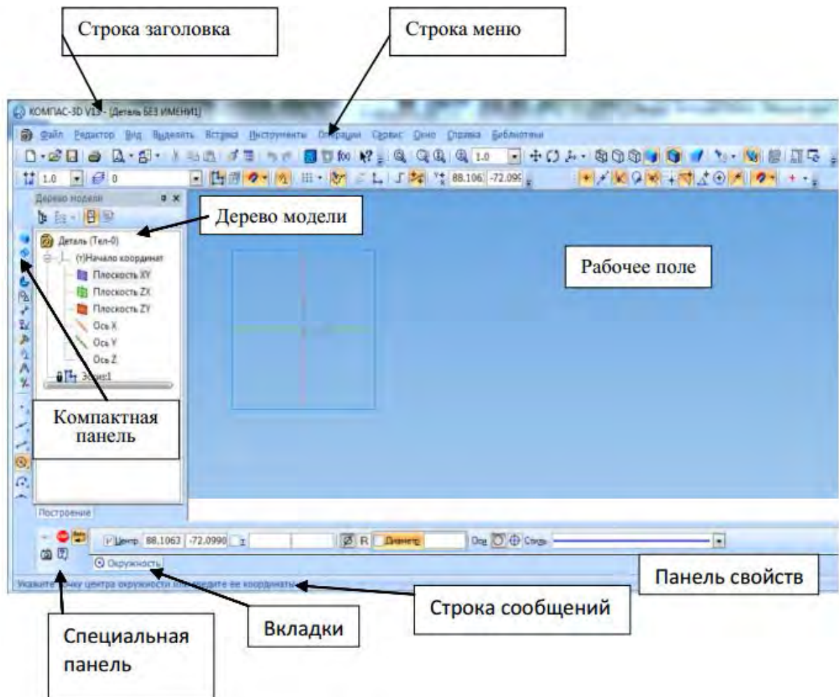
Рисунок 3.8 – Интерфейс Компас 3D
