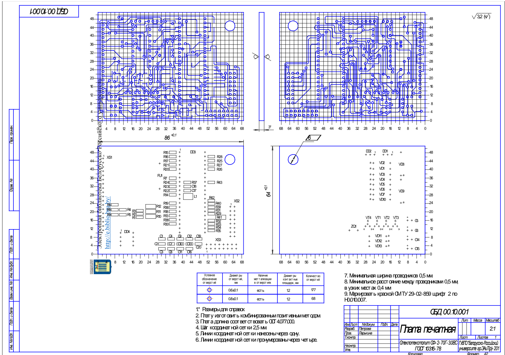
Рисунок В.10 – Пример трассировки платы печатной
