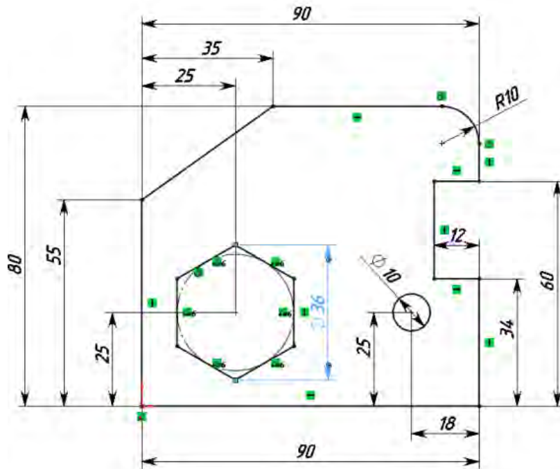
Рисунок 3.9 – Пример выполнения эскиза в среде SolidWorks
