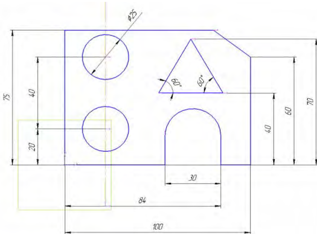
Рисунок 3.10 – Пример выполнения эскиза в среде Компас 3D
