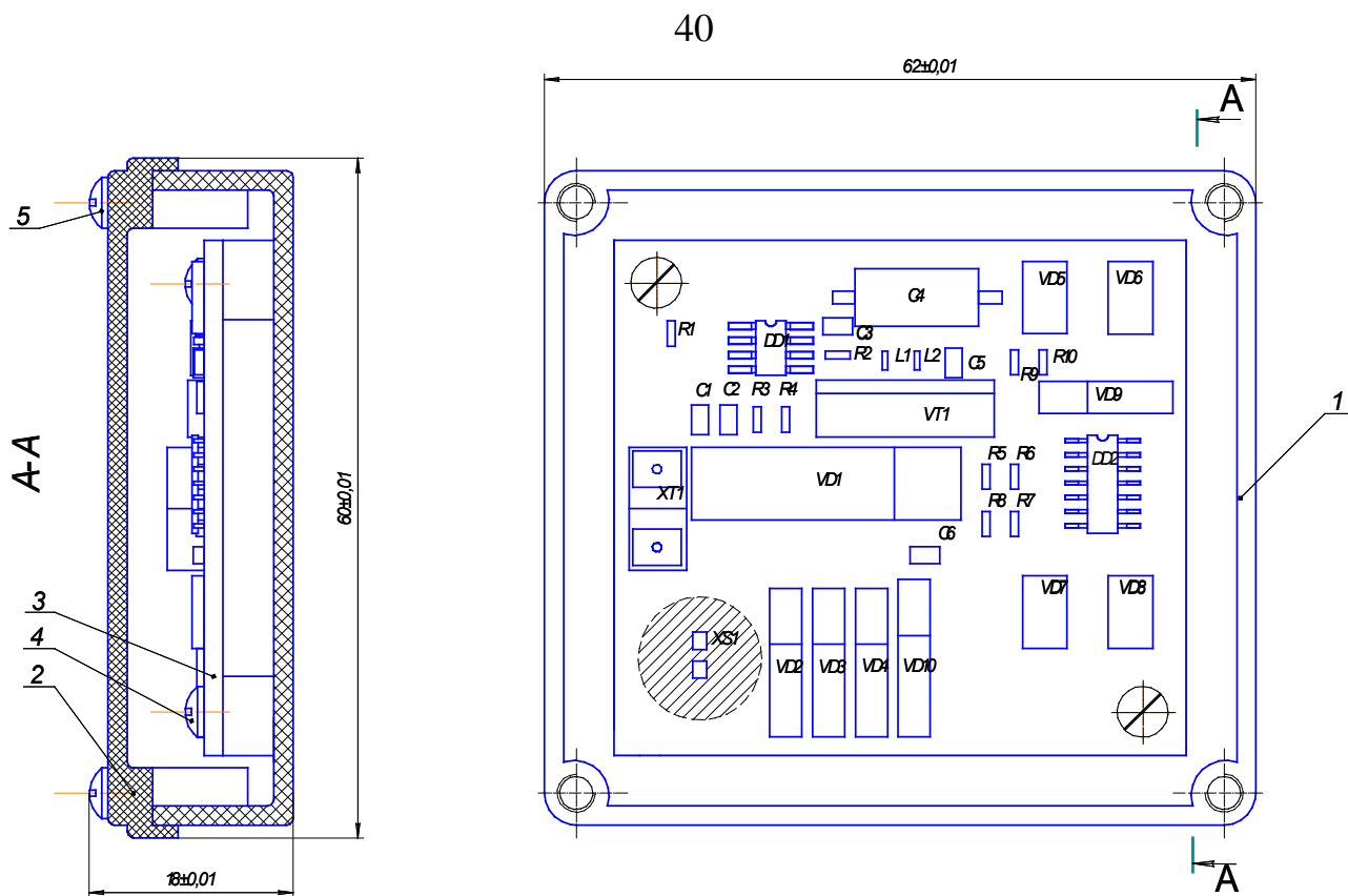
Рисунок В.5 – Пример платы печатной в сборе (с корпусом и крышкой)
