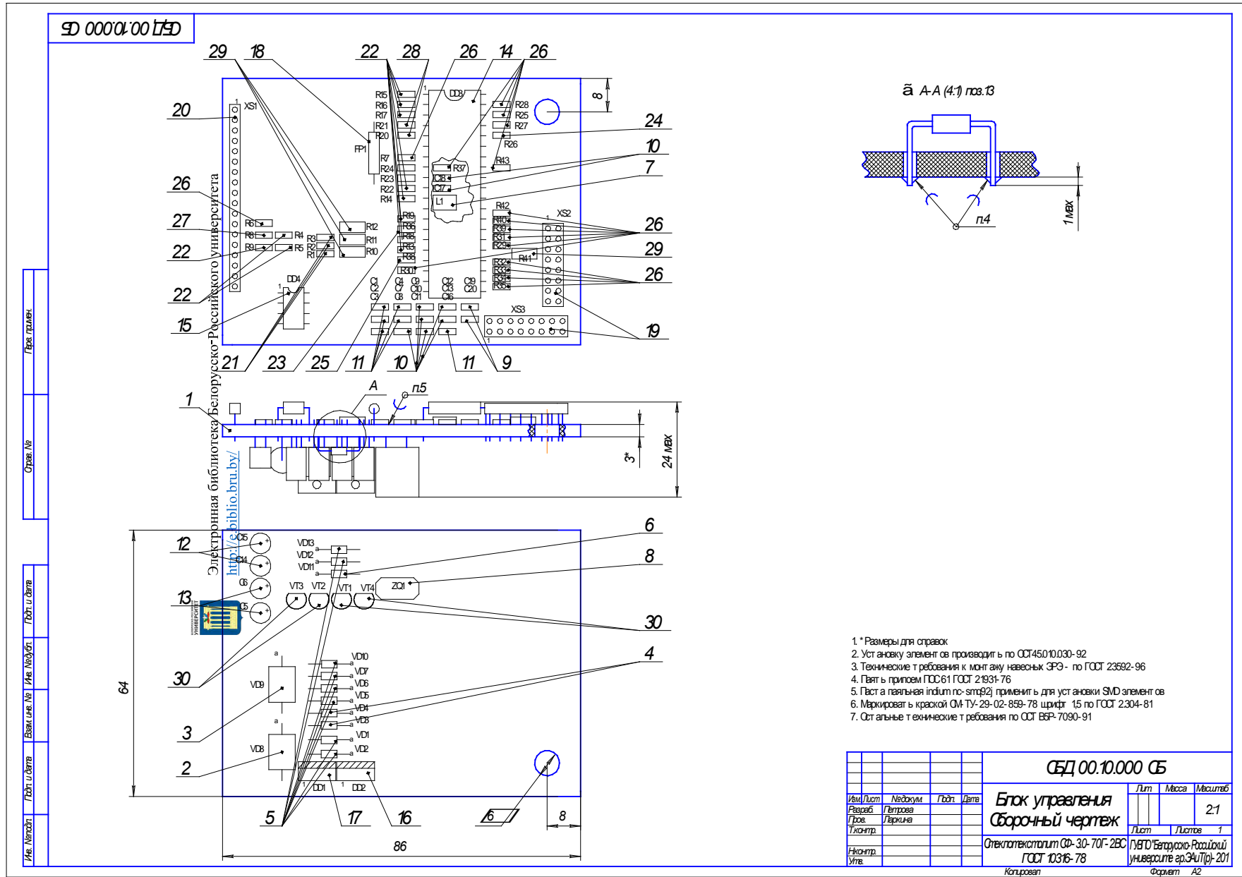
Рисунок В.9 – Пример сборочного чертежа
