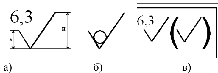
Рисунок 3.1 – Шероховатость
