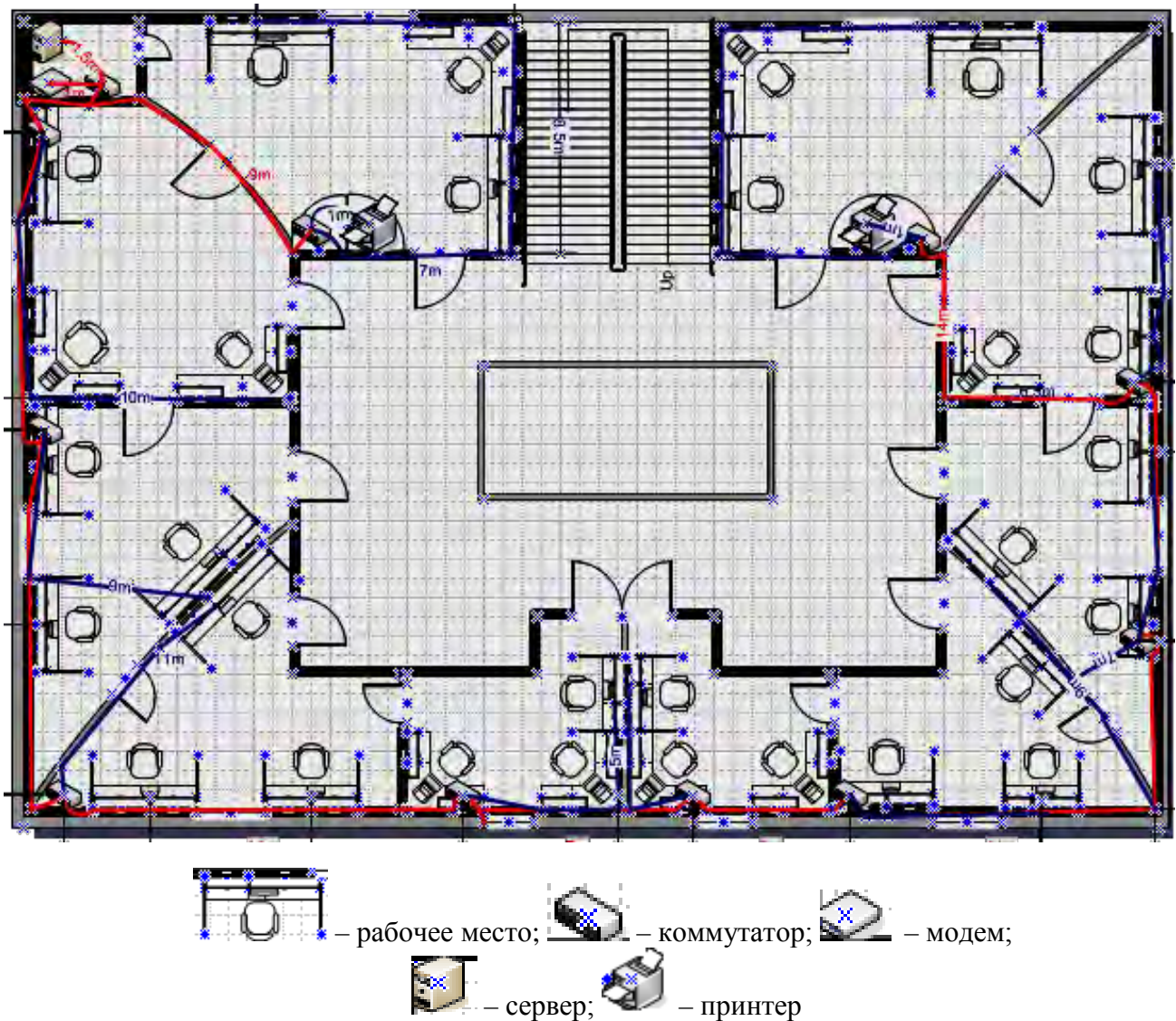
Рисунок 4 – План этажа
