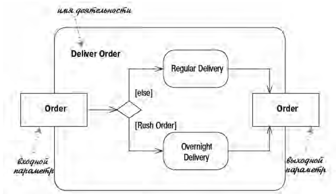
Рисунок 3 – Дополнительная диаграмма деятельности
