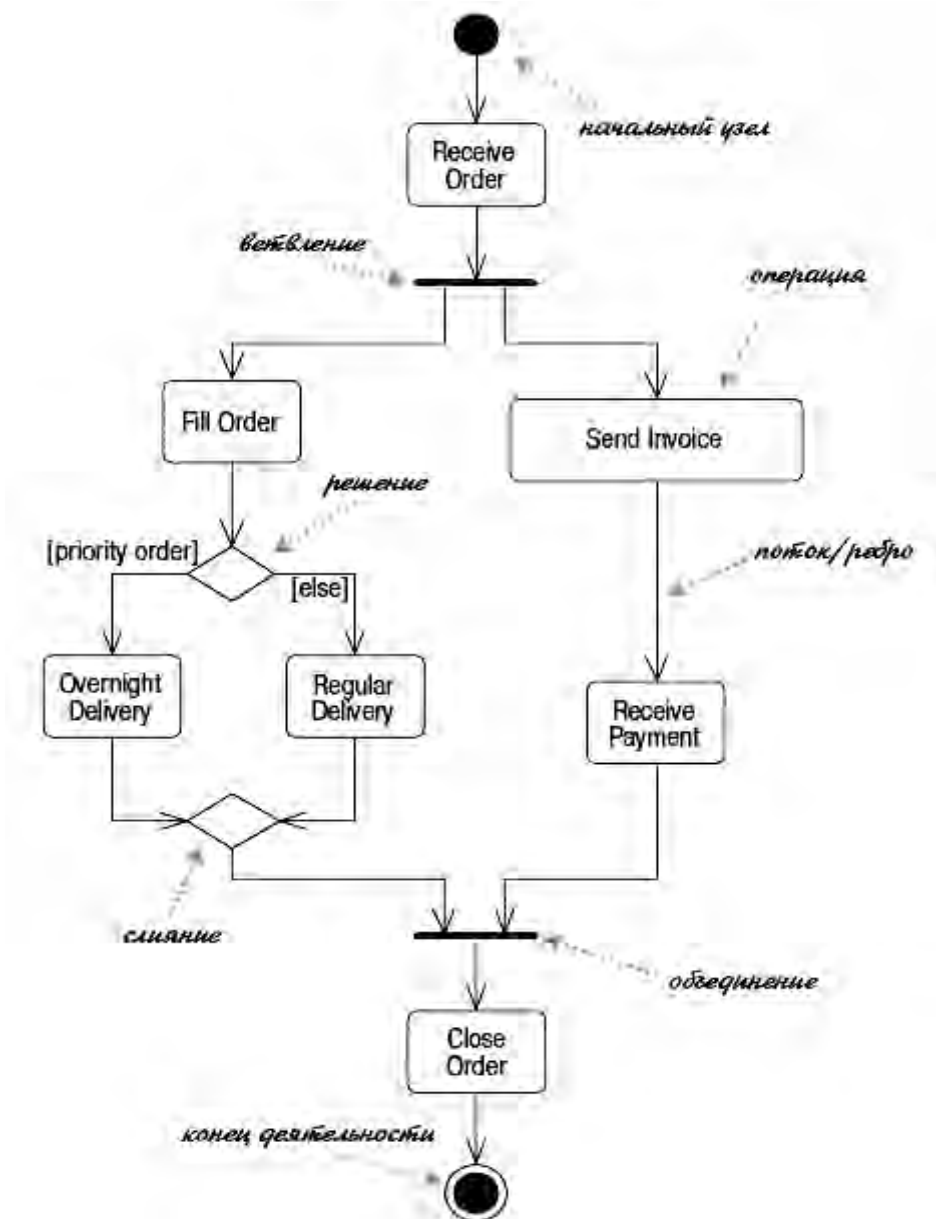
Рисунок 2 – Простая диаграмма деятельности
