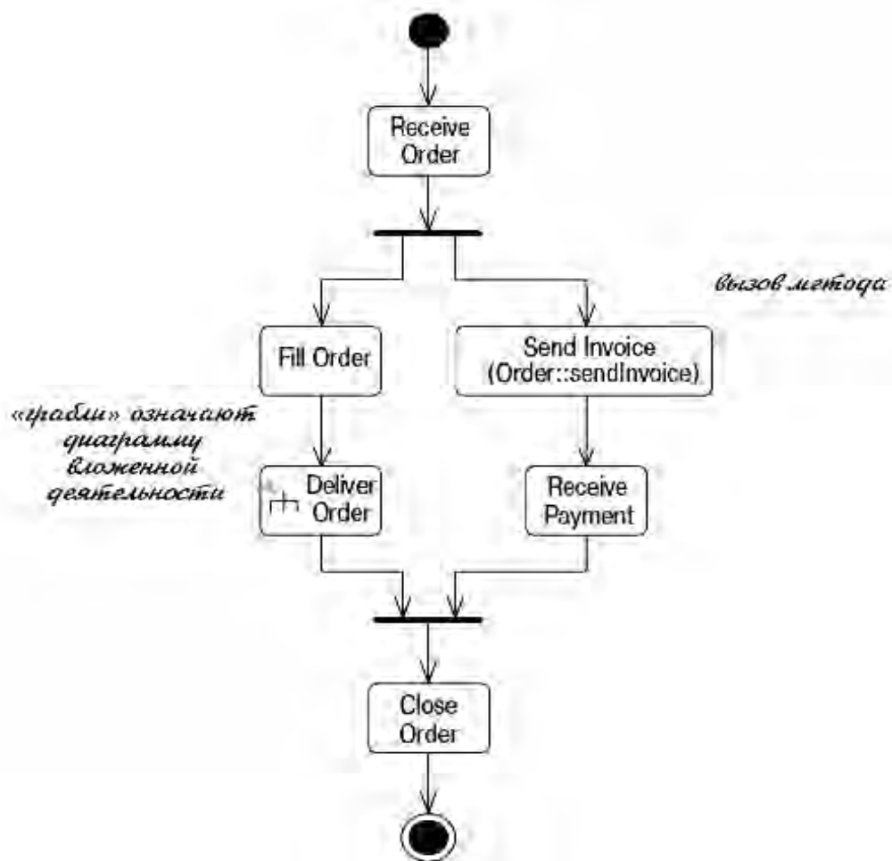
Рисунок 4 – Модифицированная диаграмма деятельности
