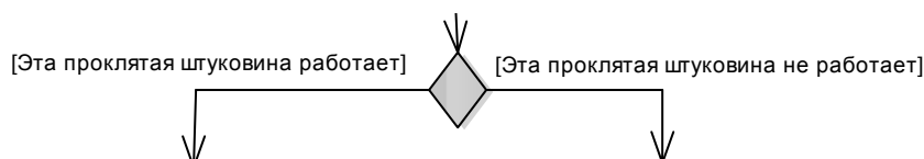
Рисунок 14 – Ветвление
