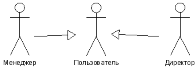
Рисунок 4 – Отношение обобщения
