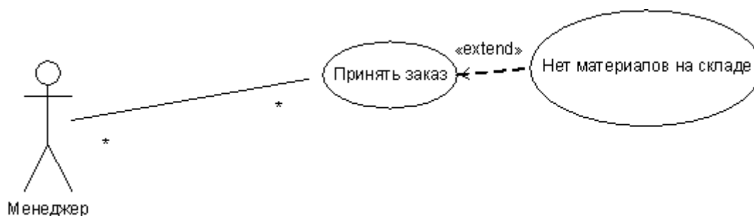
Рисунок 3 – Отношение расширения
