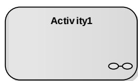
Рисунок 11 – Сложное действие
