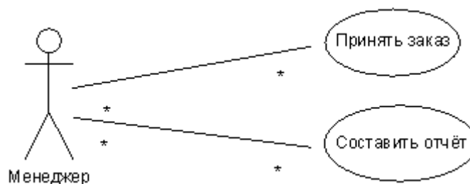
Рисунок 1 – Отношение ассоциации
