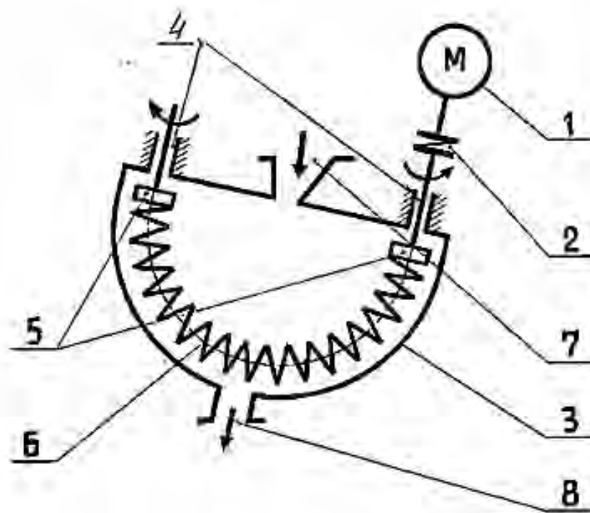
Рис. 1. Кинематическая схема пружинной мельницы
