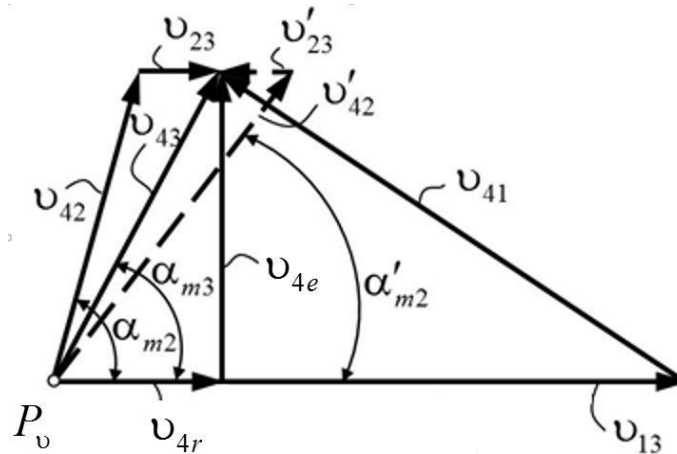
Рис. 3. План скоростей основных элементов СРП
