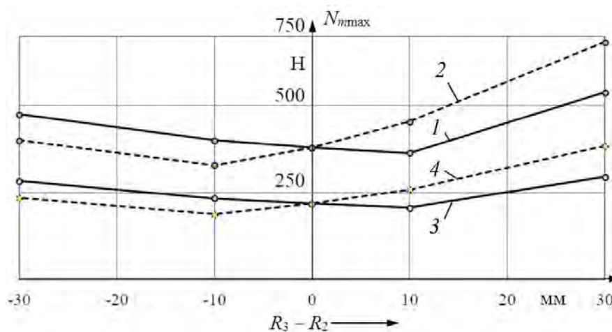
Рис. 5. Максимальные значения реакций основных звеньев СРП: 1, 2, 3 и 4 — для передач с параметрами по вариантам 1, 2, 3 и 4 (табл. 2) соответственно
