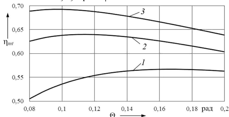
Рис. 6. Зависимость КПД роликового зацепления СРП от угла \Theta : 1, 2 и 3 – для передач с параметрами по вариантам 1, 2 и 3 (табл. 3) соответственно
