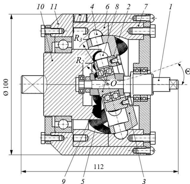
Рис. 1. Конструкция редуктора со сферической роликовой передачей
