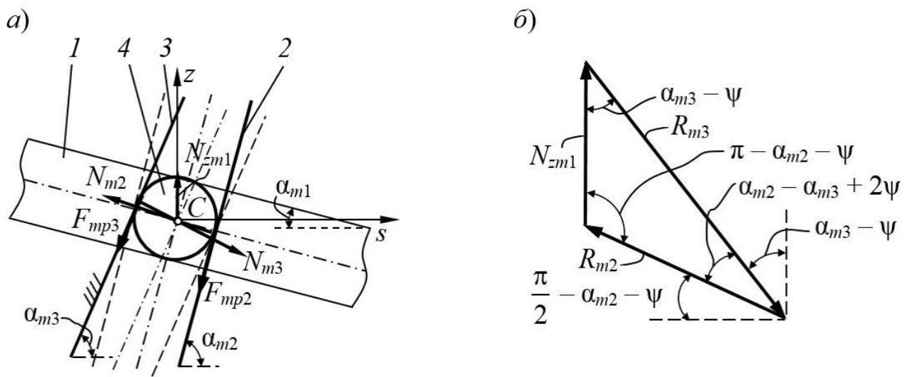
Рис. 2. К оценке сил, действующих в СРП, и КПД передачи: а – схема силового взаимодействия; б – треугольник равновесной системы сил; 1 – сателлит; 2 – кулачковая поверхность ведомого вала; 3 – неподвижная беговая дорожка; 4 – ролик
